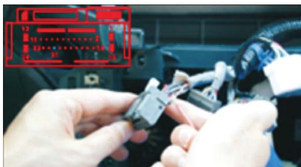
21. Подсоедините розовый провод к штатному разъему (21 pin).
