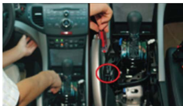
40. Установите и зафиксируйте винтами левую декоративную панель на консоли.
