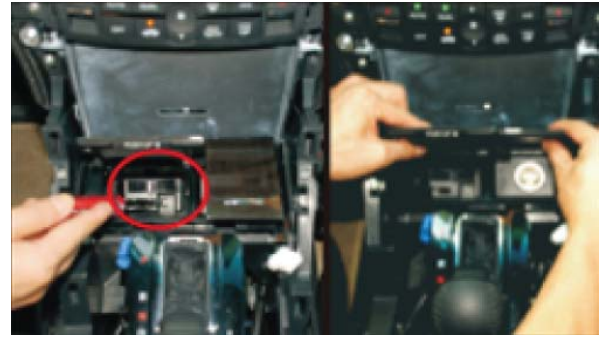
12. Демонтируйте прикуриватель с помощью отвертки, отсоедините проводку.
