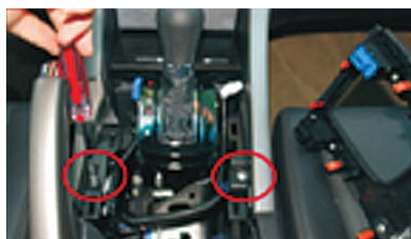
4. Открутите винты, как показано на фото.
